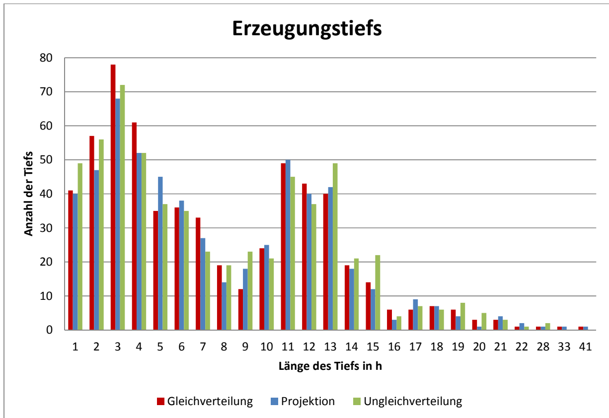
Abbildung 7: Erzeugungstiefs der kombinierten Verteilung aus Windenergie- und PV-Erzeugung (Stunden mit geringer Erzeugung kleiner gleich 10 GWh) von 2008 bis 2012:
