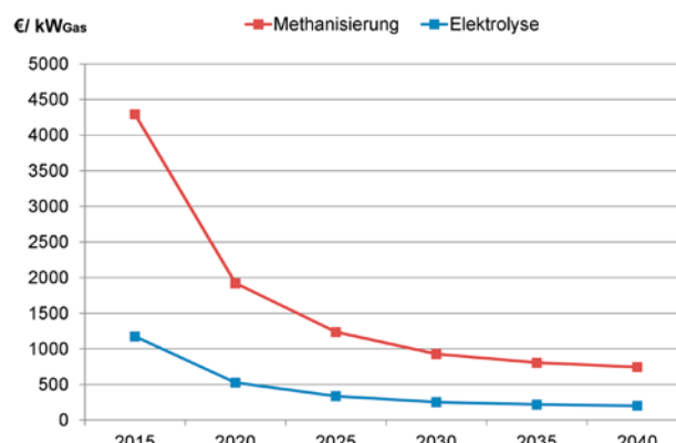
(a) Batteriespeicher (b) Power-to-Gas-Komponenten Abbildung 13: Angenommene Investitionskosten für Speichertechnologien
